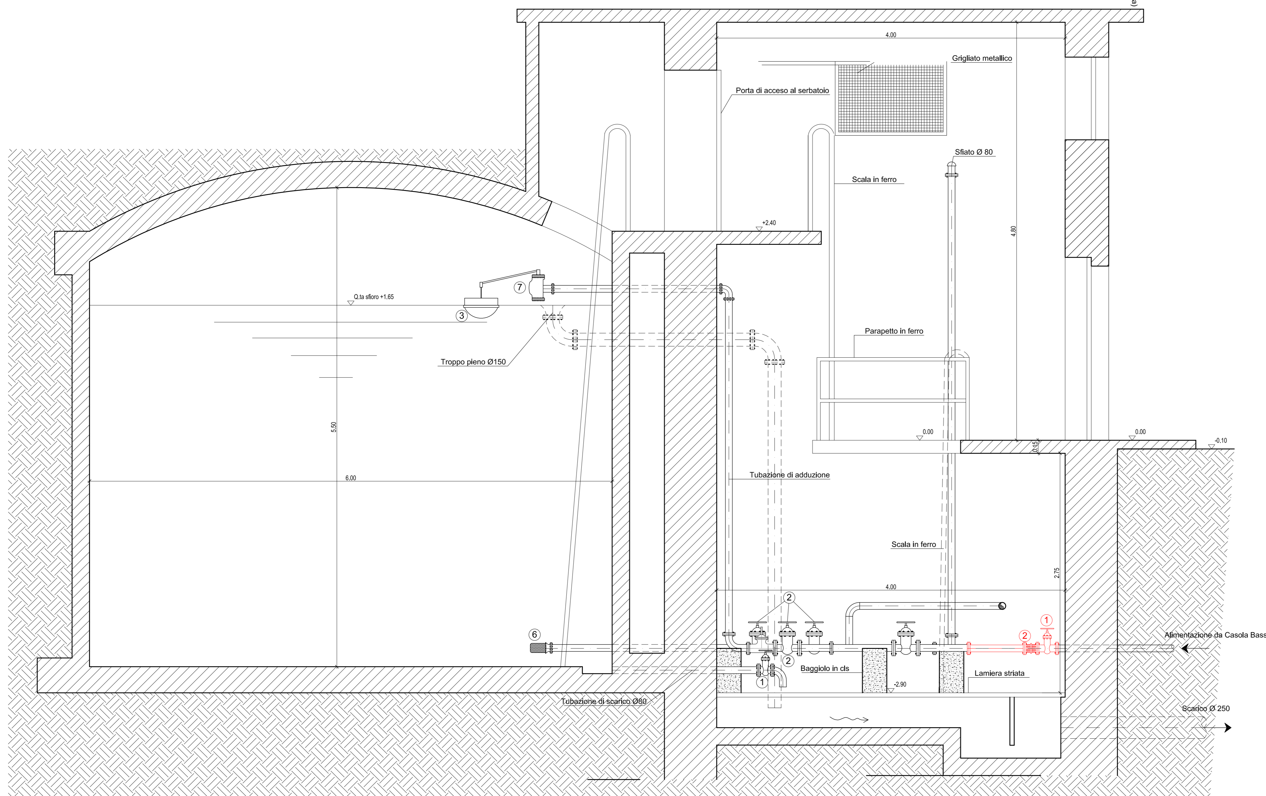
SEZIONE B - B SCALA 1:25
