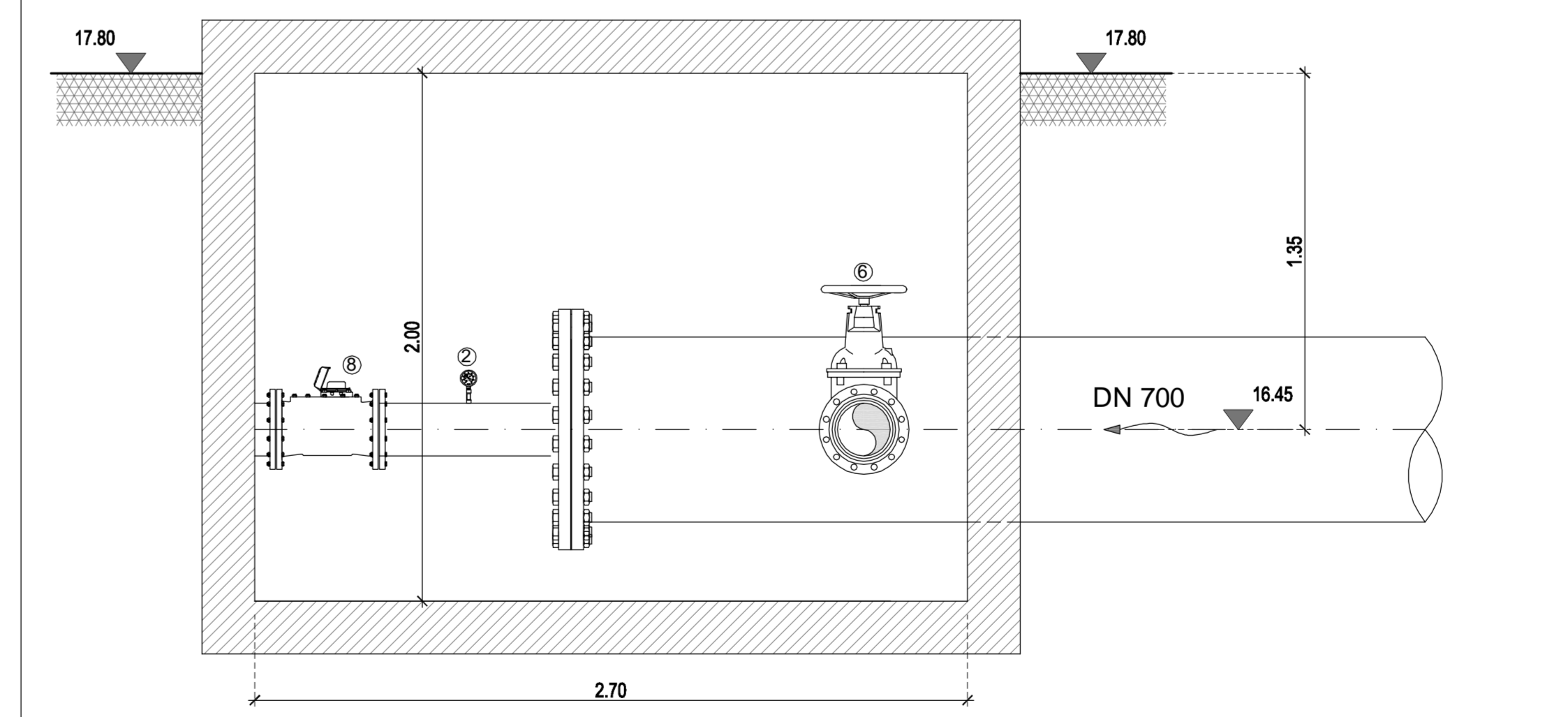
SEZIONE A - A Scala 1:20
